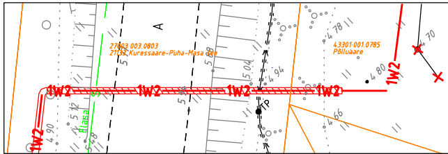
21133 Kuressaare-Puha-Masa tee (27003 003 0803) Maantee alt kinnine labidamine km-l 7,23
