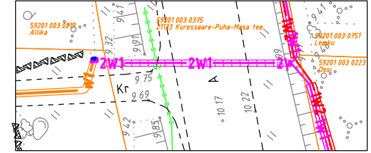
21133 Kuressaare-Puha-Masa tee (59201 003 0375) Maantee alt kinnine labidamine km-l 11,41
