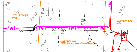
21133 Kuressaare-Puha-Masa tee (27003 003 0803) Maantee alt kinnine labidamine km-l 11,08
