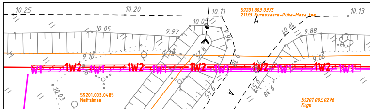
Kiige (59201 003 0276) ja Neitsimäe (59201 003 0485) Sõidutee ja kraavi alt kinnine labidamine
